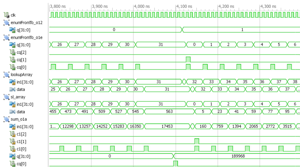
4.17. ábra. SFB szimuláció, ssom fokozat (nagyfelbontás)
