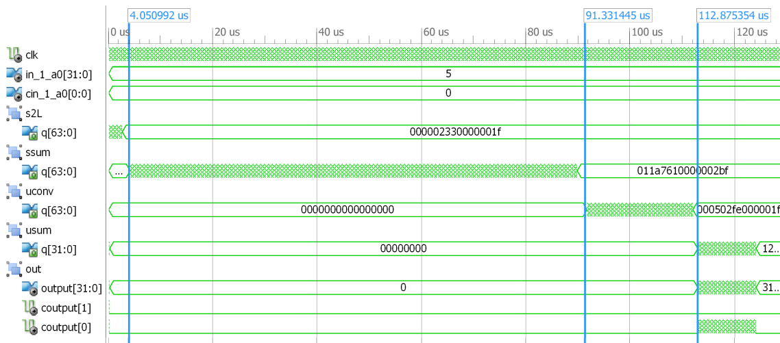
4.15. ábra. SFB modul full
