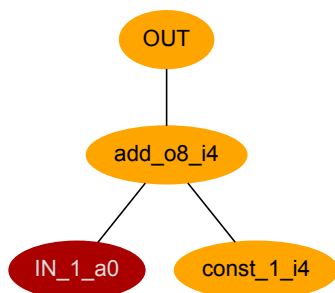
2.11. ábra. OpTree
